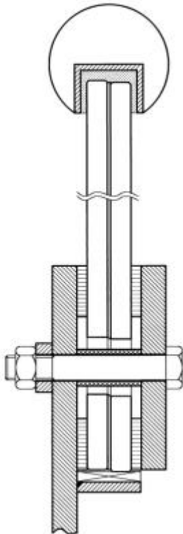
Prinzipskizze
